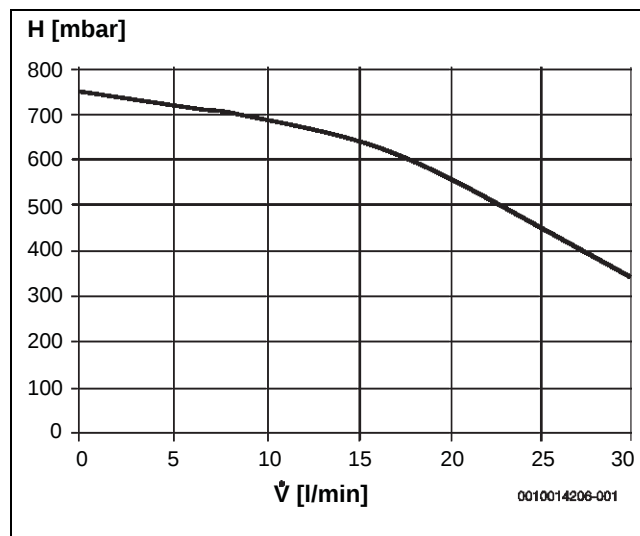
Bild 215 Restförderdruck Primärseite
