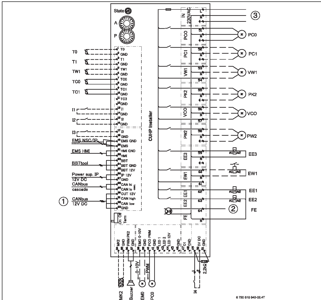
Bild 157 Schaltplan Installationsmodul integrierter elektrischer Zuheizer
