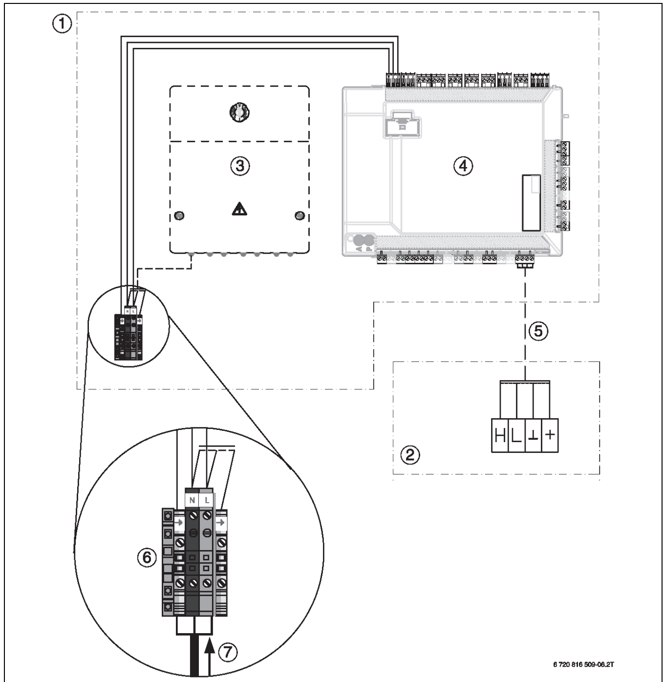
Bild 164 Inneneinheit mit externem Zuheizer – Überblick
