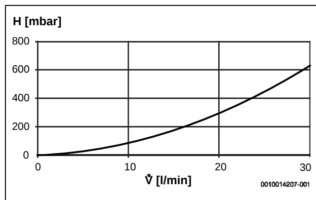
Bild 216 Druckverlust Sekundärseite
