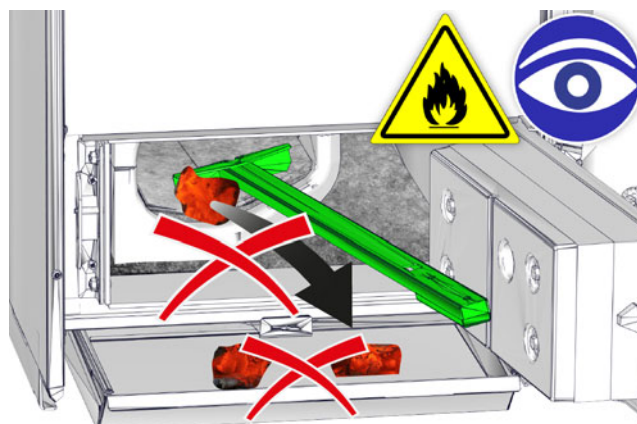
Sl. 6-4: V predal za pepel ne vnašajte žerjavice
