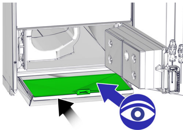
Sl. 6-8: Pokrov predala za pepel
