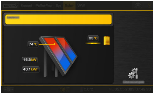
Sl. 7-111: Solarna naprava z zunanjim izmenjevalnikom toplote in ventilom za slojno polnjenje
