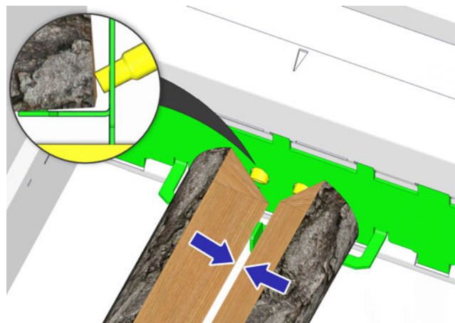
Sl. 6-21: Polena na nastavku za prižiganje
