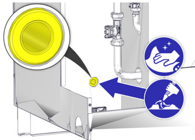
Sl. 10-3: Ležišče tesnila lambda sonde
