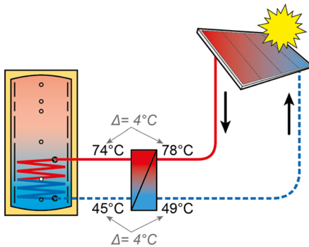
Sl. 7-110: Princip regulacije
