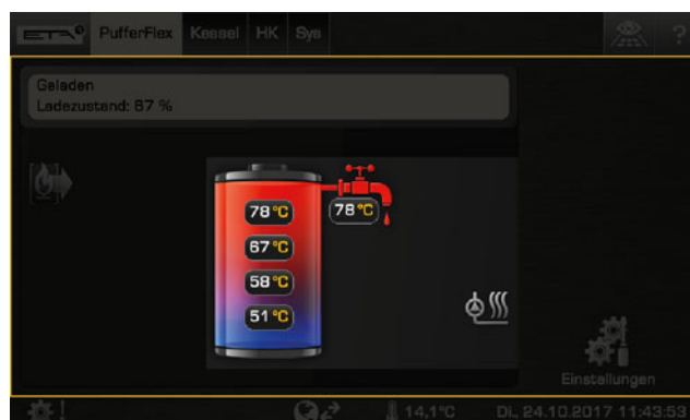
Sl. 7-84: Kombiniran zalogovnik
