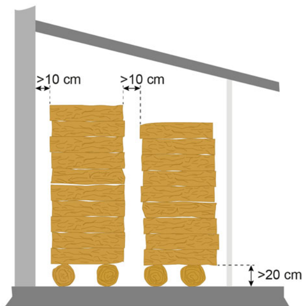
Sl. 4-4: zaščiteno mesto za skladiščenje ob steni objekta
