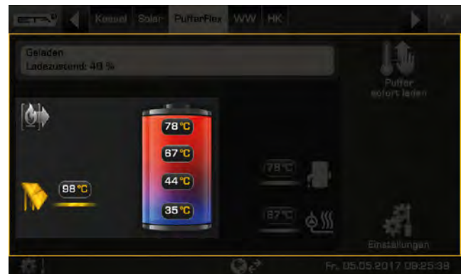
Sl. 5-54: Solarna naprava na vmesnem zbiralniku
