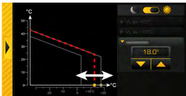
Sl. 5-72: Meja gretja za način ogrevanja
