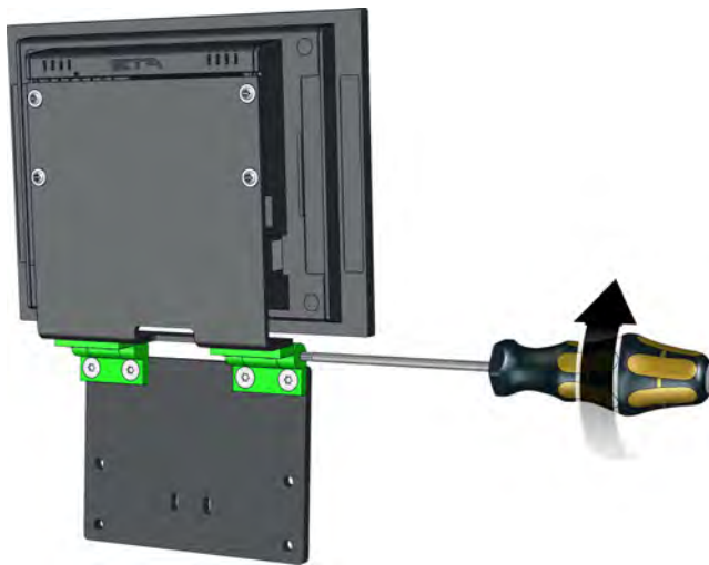
Sl. 2-5: Tečaji
