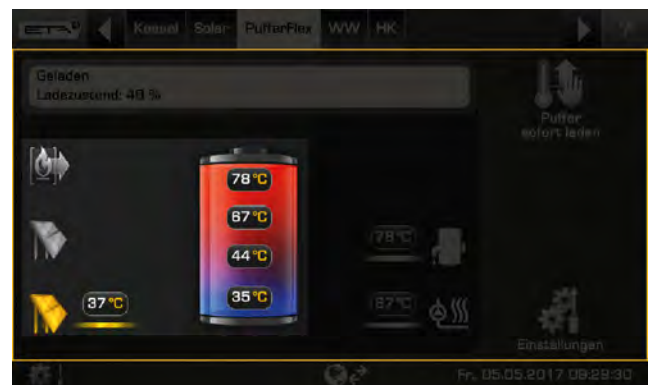
Sl. 5-55: Slojno polnjenje vmesnega zbiralnika
