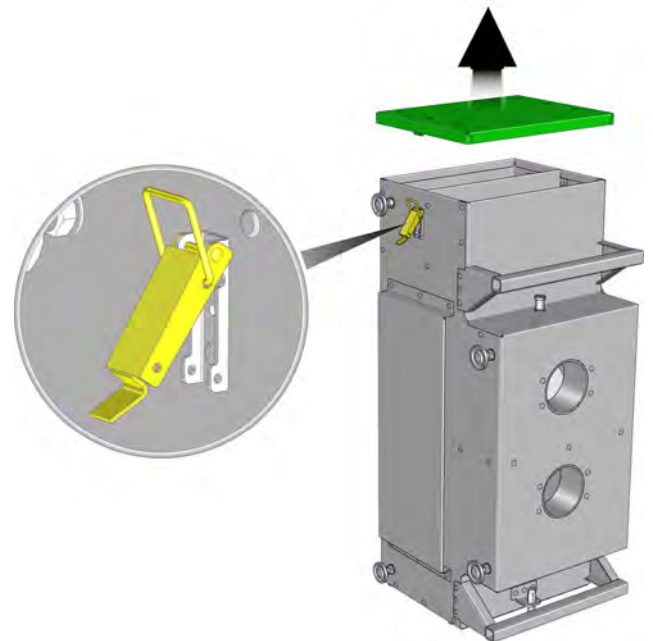
Sl. 4-2: Pokrov
