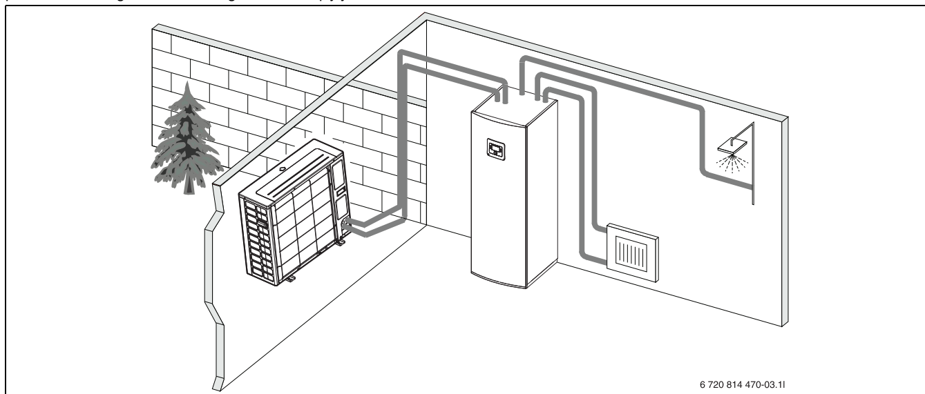
Sl.2 Zunanja enota toplotne črpalke, notranja enota AWMS/AWMSS z vgrajenim boilerjem in električnim grelnikom
