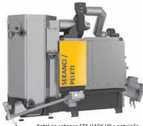
Kotel na sekance ETA HACK VR s potujočo rešetko, 250 - 333 - 350 - 500 kW
