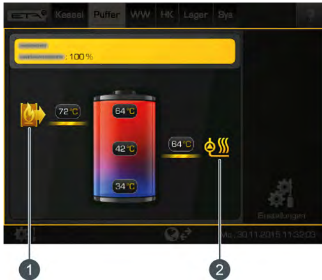
Sl. 6-21: Pregled porabnika in generatorja
