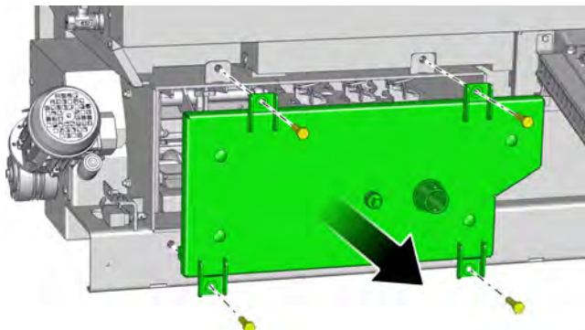
Sl. 8-22: Vzdrževalni pokrov
