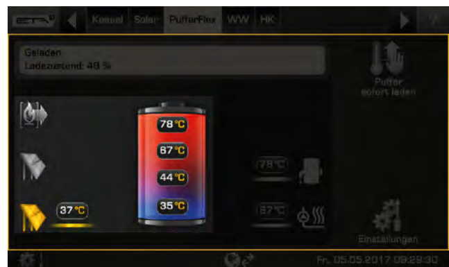
Sl. 6-51: Slojno polnjenje vmesnega zbiralnika
