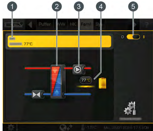
Sl. 6-79: Daljinsko ogrevanje kot predajna postaja
