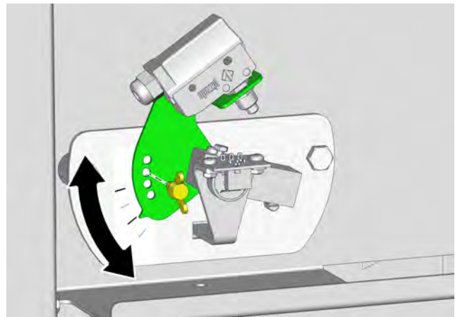
Sl. 4-3: Nastavljivo nivojsko stikalo žerjavice
