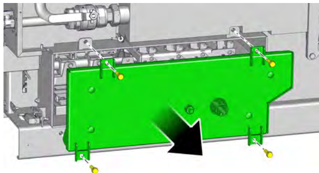
Sl. 8-24: Vzdrževalni pokrov
