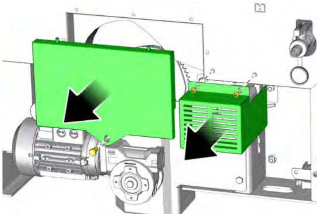
Sl. 8-12: Pokrovi
