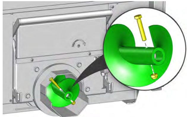
Sl. 8-4: Odstranjevanje vijaka
