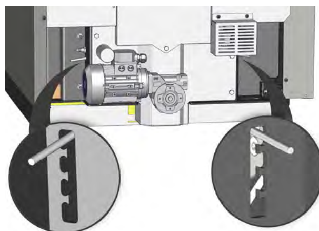
Sl. 2-6: Vzvod
