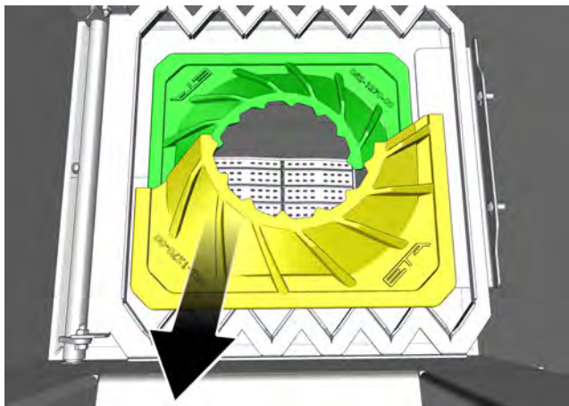
Sl. 8-7: Odstranjevanje pokrova zgorevalne komore
