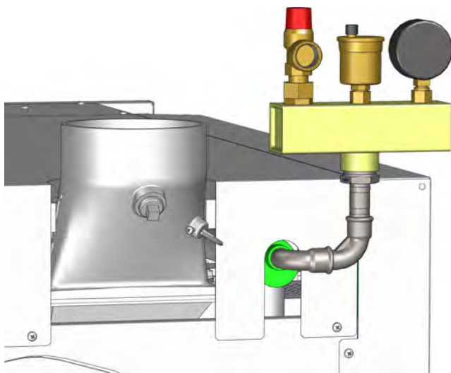
Sl. 3-5: Priključek
