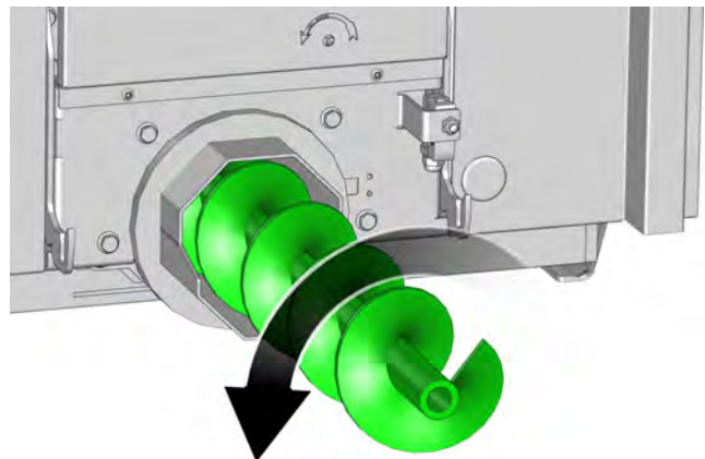
Sl. 8-5: Odvijanje polža za pepel
