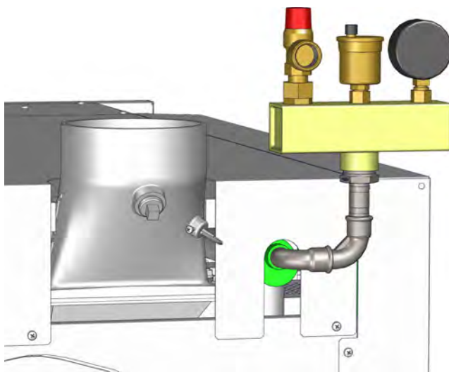
Sl. 3-5: Priključek
