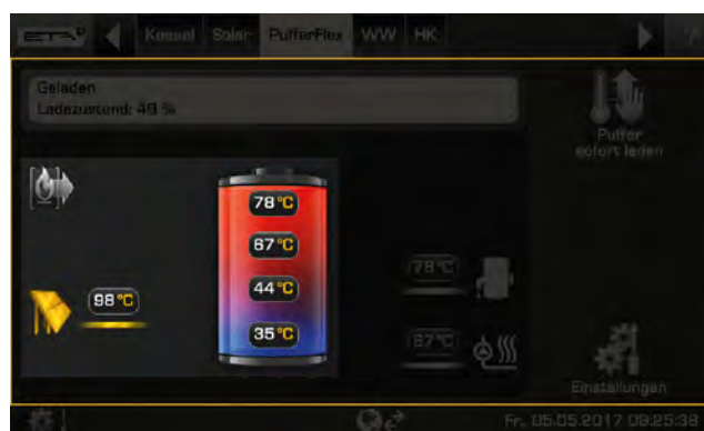
Sl. 5-50: Solarna naprava na vmesnem zbiralniku
