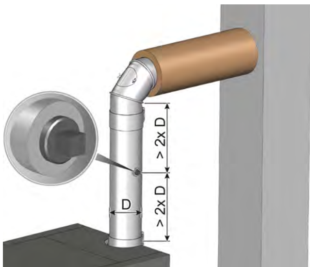
Sl. 6-1: Razdalje za merilno odprtino
