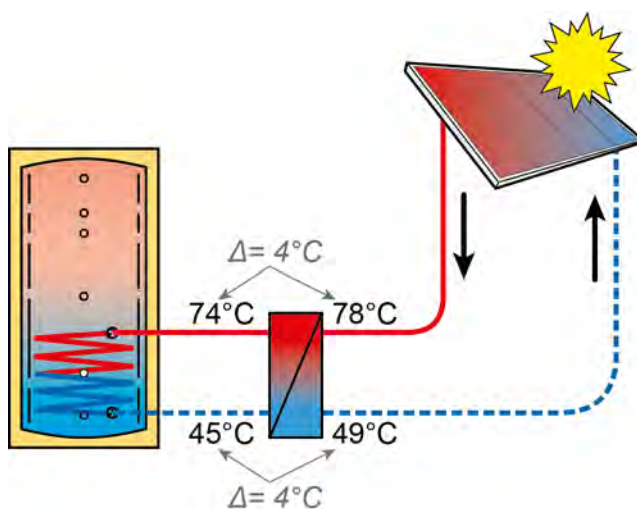
Sl. 5-74: Princip regulacije
